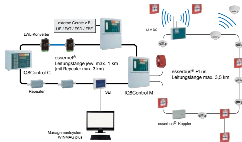
Anschaltungsbeispiel
