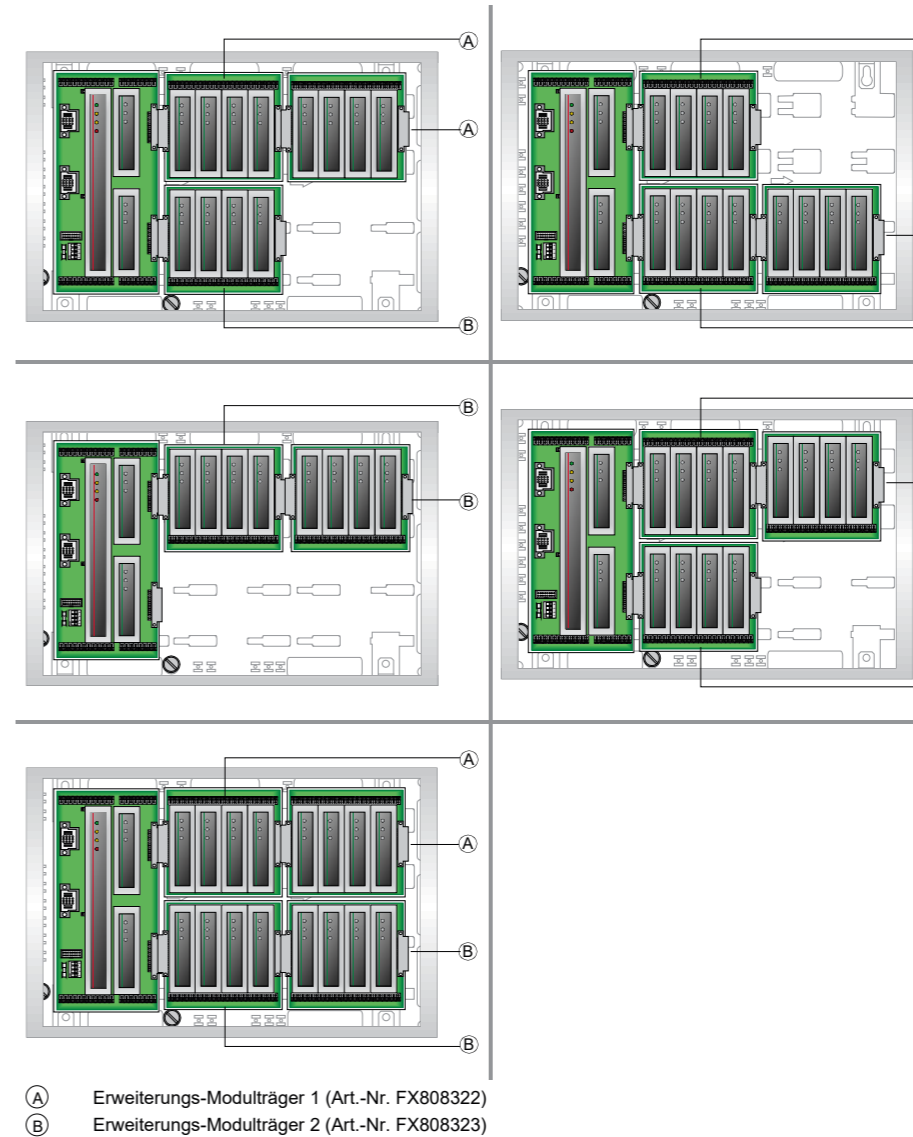
Variabler Einbau der Erweiterungs-Modulträger (senkrechter Einbau mit Rückwand Art.-Nr. FX808311)
