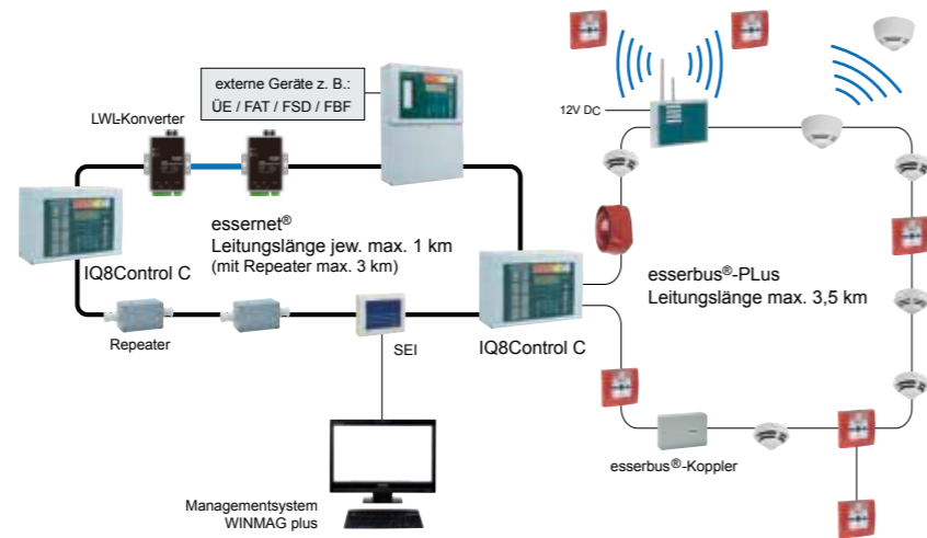
Anschaltungsbeispiel
