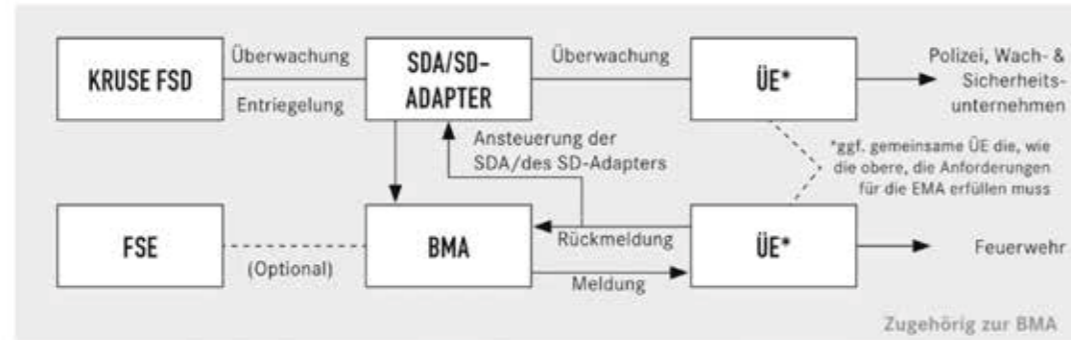
Anschaltbeispiel „A“
