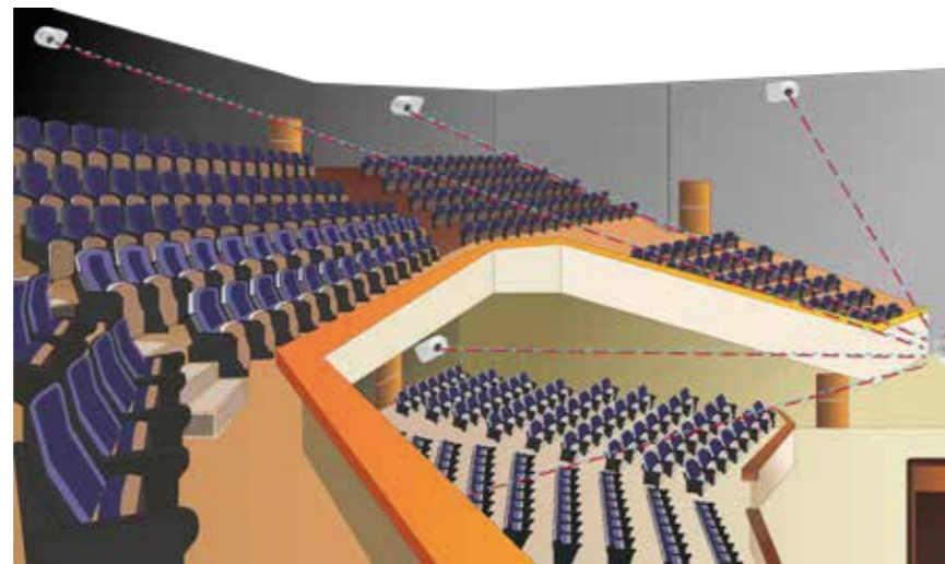
Anwendungsbeispiel mit fünf Sendern/Lichtquellen OSE-xy und und einem OSID Empfänger OSI-90
