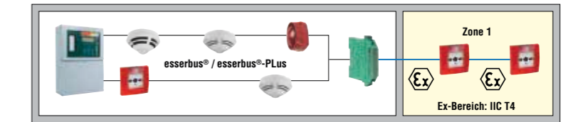
Ex-Barriere (Art.-Nr. 804744)
