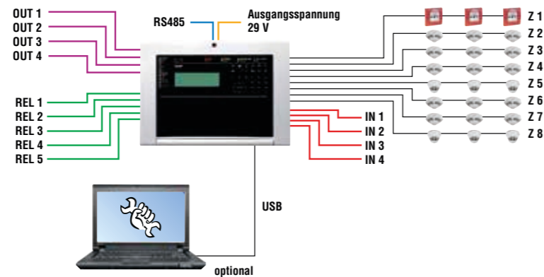
Anschaltungsbeispiel
