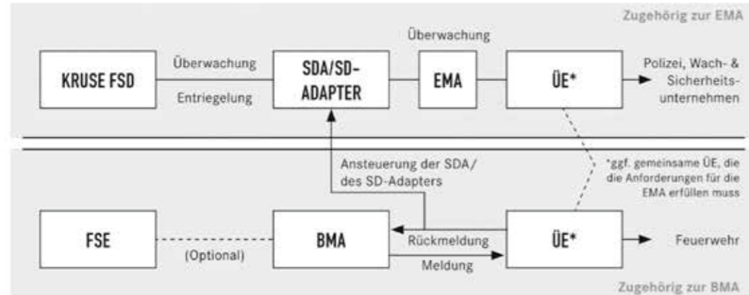
Anschaltbeispiel „B“
