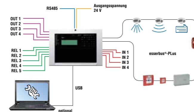
Anschaltungsbeispiel
