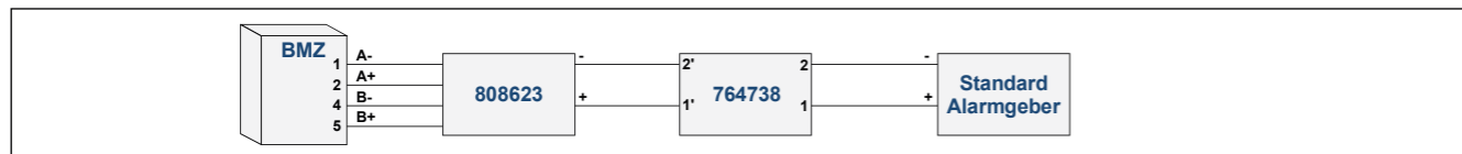
ÜSS-Modul 764738 mit esserbus®-Alarmierungskoppler 808623 und Standard Alarmgeber
