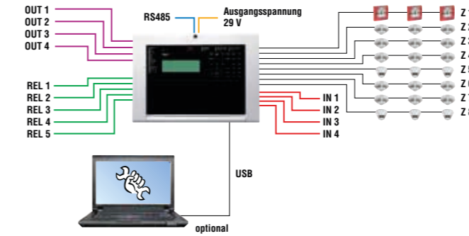
Anschaltungsbeispiel
