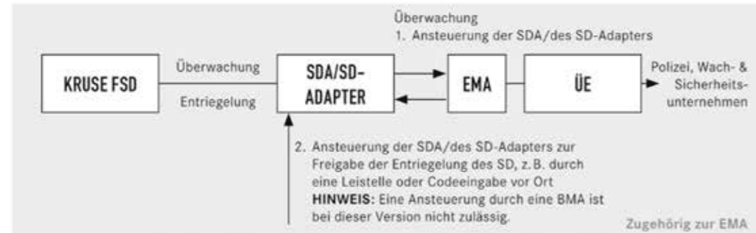
Anschaltbeispiel „C“
