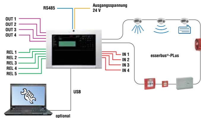
Anschaltungsbeispiel
